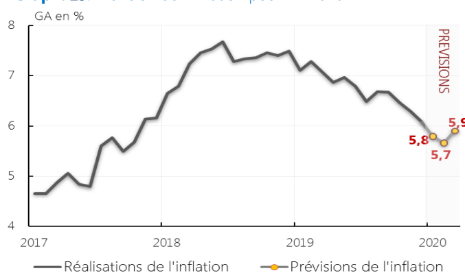
Graph. 23: Prévision de l'inflation pour T1-2020
